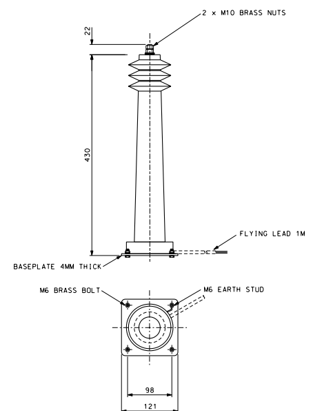
EC3239 Dimensions
